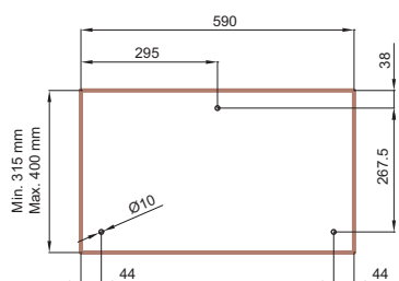
T-bracket ( LTTABTB )
