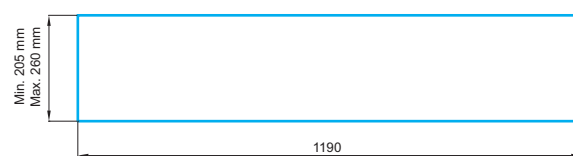
200-mm shelf bracket ( LTTAB20V )
