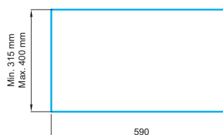
T-bracket ( LTTABTV )
